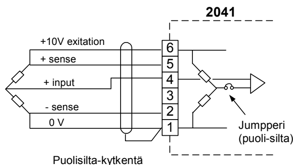
Puolisilta-kytkentä
